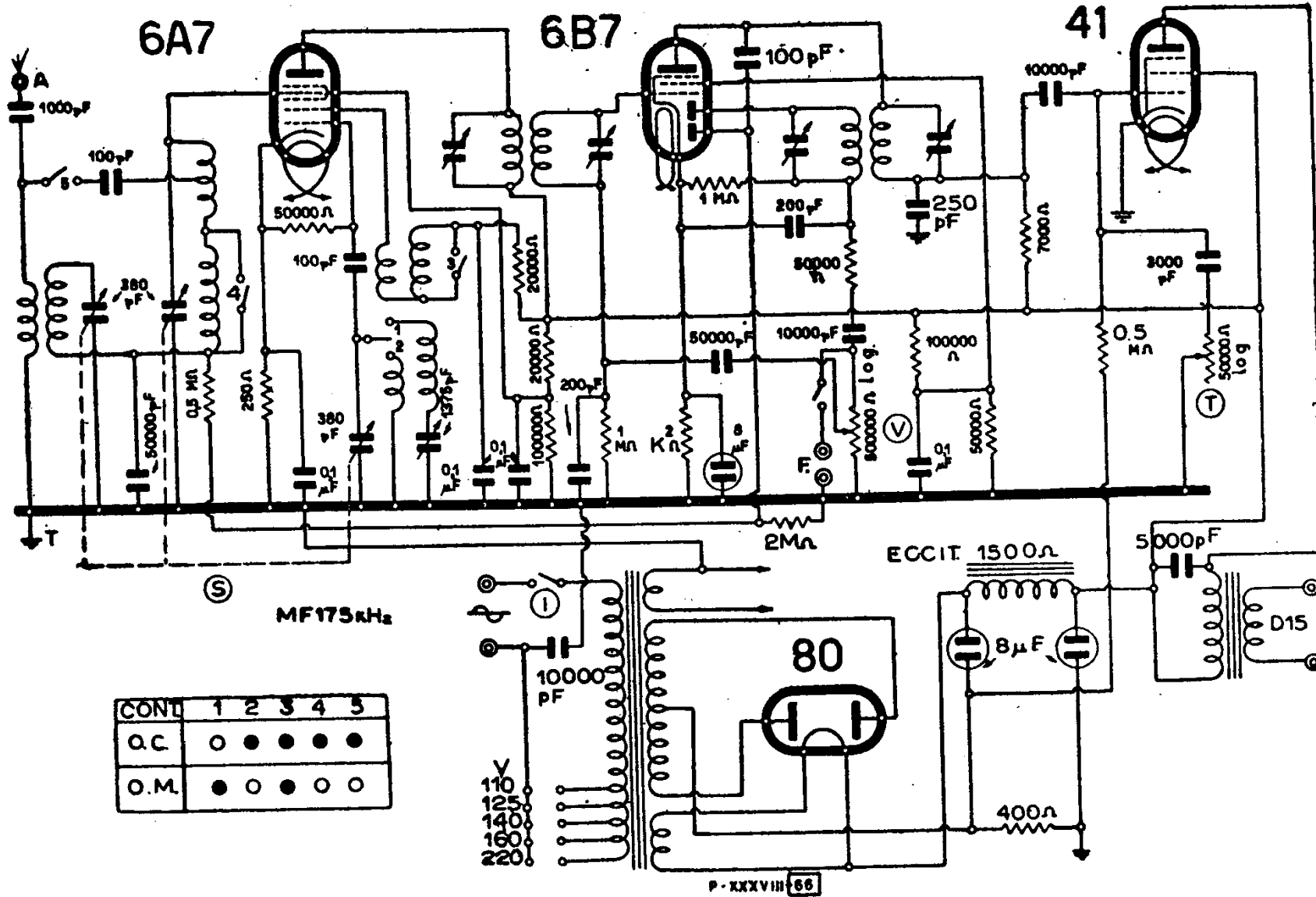
WATT RADIO - MOD. « ONDINA IV »
